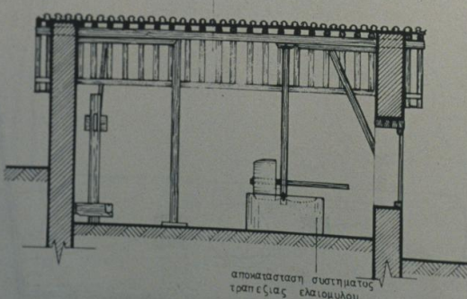
10. Ελιόμυλος στα Σπήλια, επαρχία Λευκωσίας. Κάτοψη, τομή ΑΑ και τομή ΒΒ.
